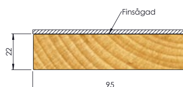
Klädسل 22 × 95 mm
